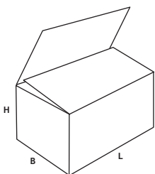
FEFCO 0703 Vouwdoos met volledig overlappende auto-lock bodem
