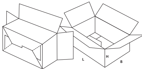
FEFCO 0711 Vouwdoos met auto-lock bodem en afdekkleppen
