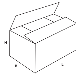
FEFCO 0701 Vouwdoos met volledig overlappende auto-lock bodem
