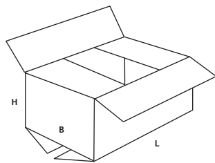
FEFCO 0711 Vouwdoos met auto-lock bodem en afdekkleppen
